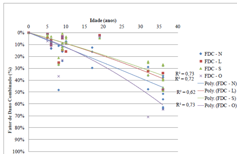
Figura 13 – Curvas de degradação em função da orientação para o Fator de Danos Combinado
