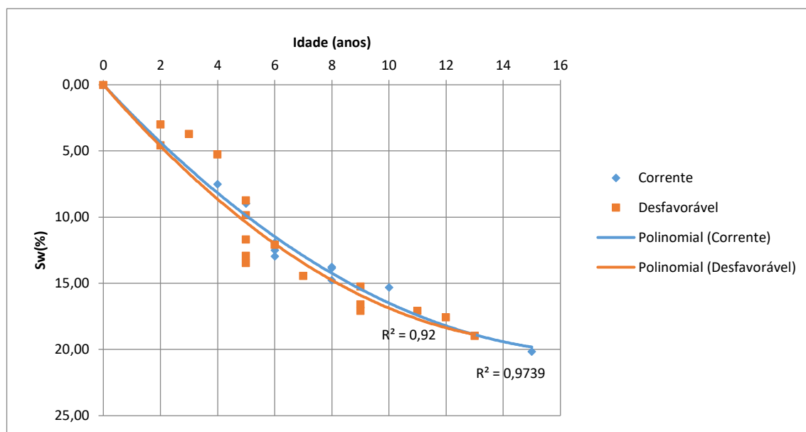
Figura 55 - Curvas de degradação dos edifícios em função da proximidade de fontes poluentes
