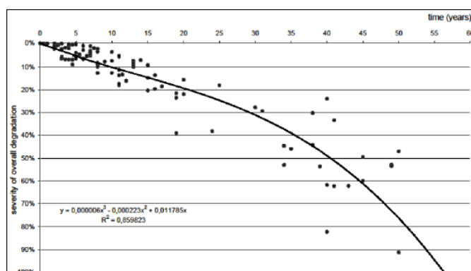
Figura 8 – Curva de degradação média de 100 amostras, expressando o NGD ao longo do tempo
