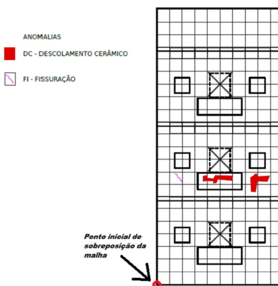
Figura 17 – Esquema ilustrativo de sobreposição da malha
