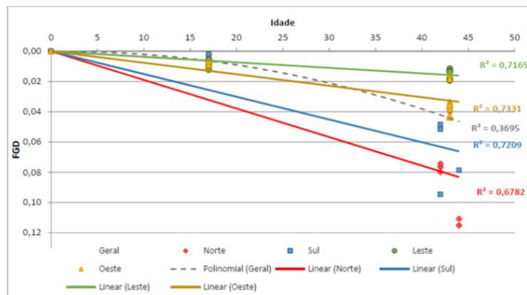
Figura 16 - Comportamento da degradação para diferentes orientações ao longo do tempo (FGD x Idade)
