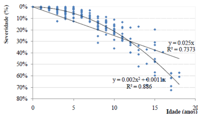
Figura 11 - Curvas de degradação (linear e polinomial) obtidas a partir dos 220 estudos de caso
