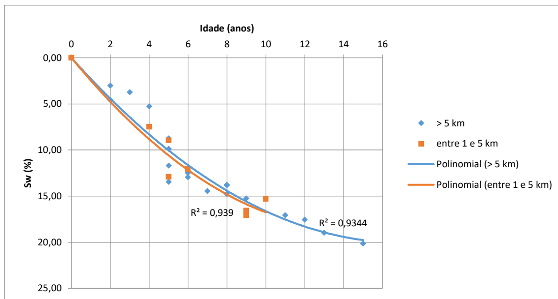
Figura 53 - Curvas de degradação dos edifícios em função da distância do mar
