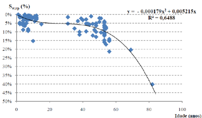
Figura 10 – Curva de degradação dos revestimentos pétreos de fachada obtida a partir de cento e vinte casos analisados no trabalho de campo
