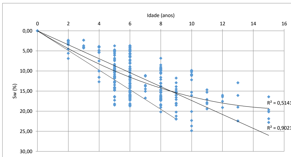
Figura 44 – Curvas de degradação (linear e polinomial) das 236 fachadas analisadas
