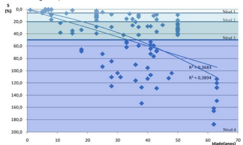
Figura 9 – Curvas de degradação de 117 amostras de revestimento cerâmico de fachada de Portugal
