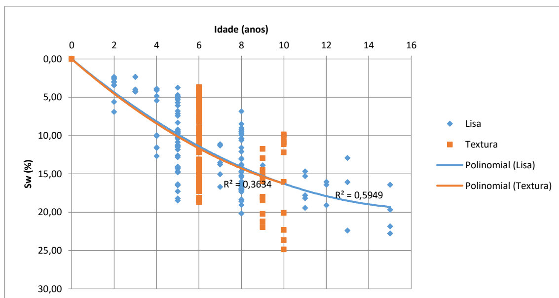
Figura 48 - Curvas de degradação das fachadas em função da textura
