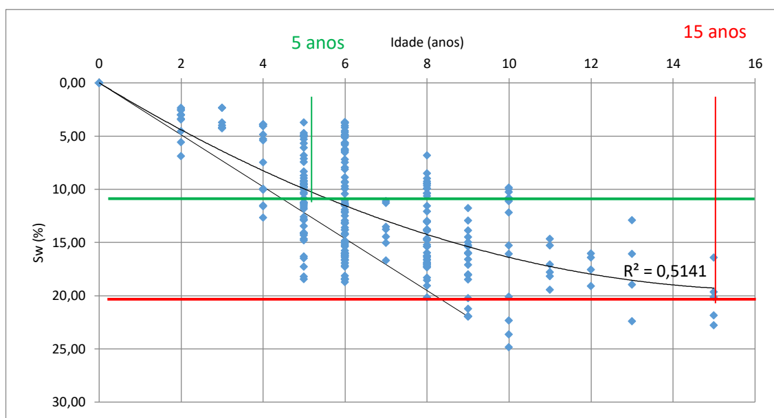
Figura 57 – Curvas de degradação (regressão polinomial) das 236 fachadas analisadas
