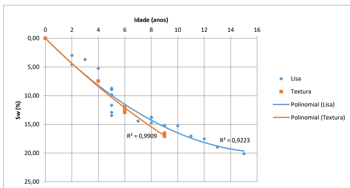
Figura 49 - Curvas de degradação dos edifícios em função da textura
