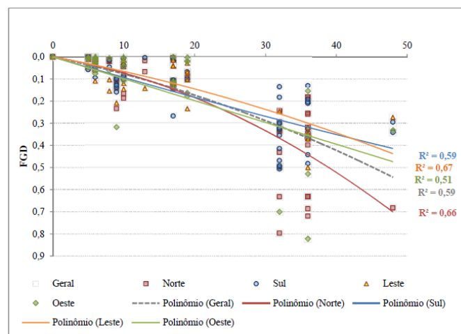
Figura 15 – Curvas de degradação em função da orientação para o Fator Geral de Danos em relação do tempo
