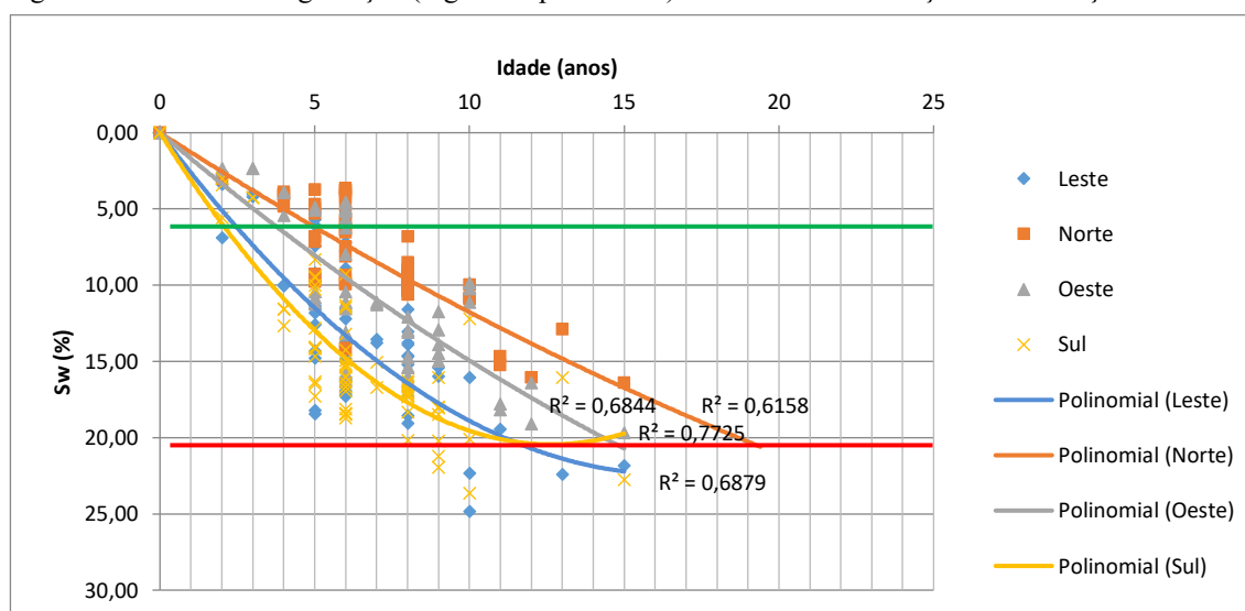
Figura 59 - Curvas de degradação (regressão polinomial) das fachadas em função da orientação cardinal
