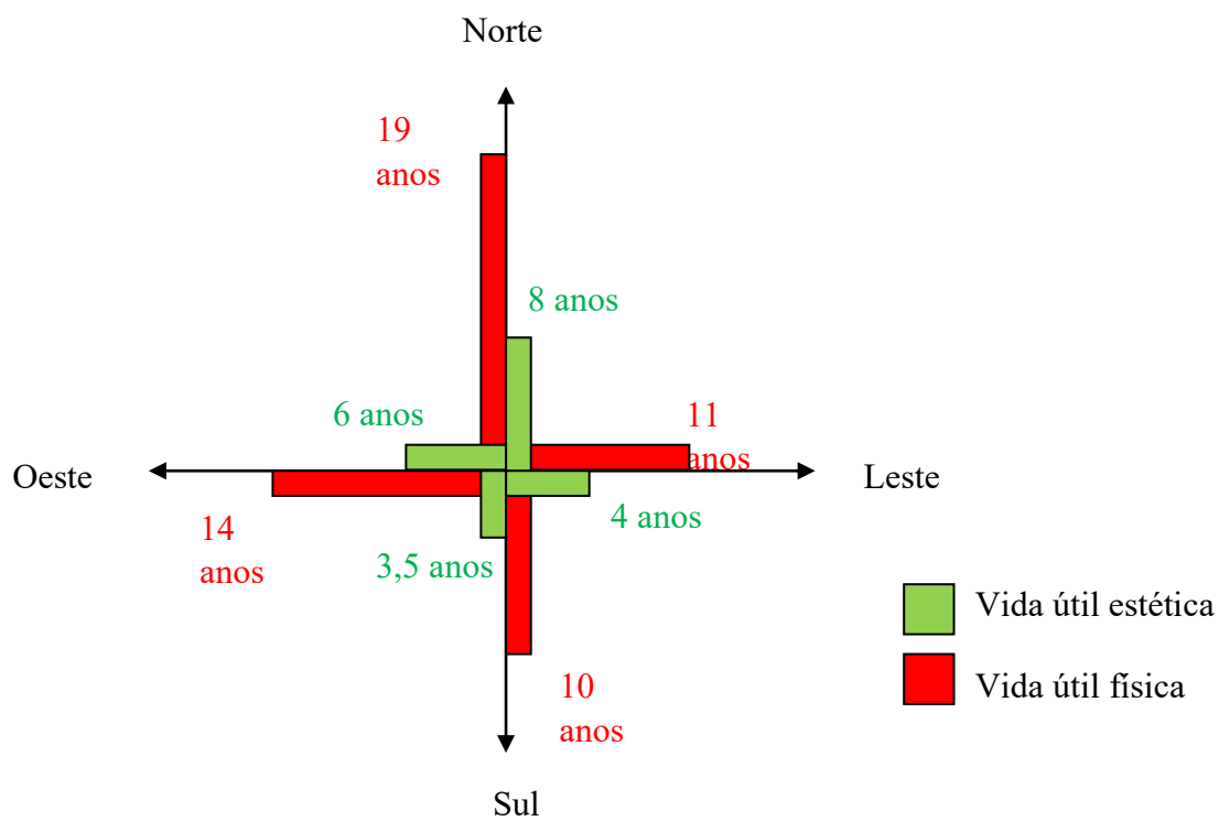
Figura 60 – “A cruz da vida útil”: vidas úteis em função da orientação cardeal
