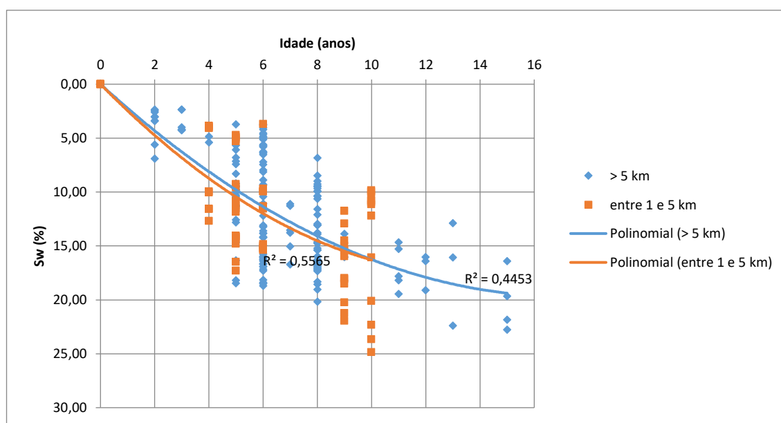
Figura 52 - Curvas de degradação das fachadas em função da distância do mar
