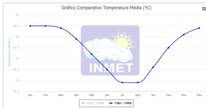
Figura 25 – Gráfico Climatológico da temperatura média de Recife – período de 1961-1990
