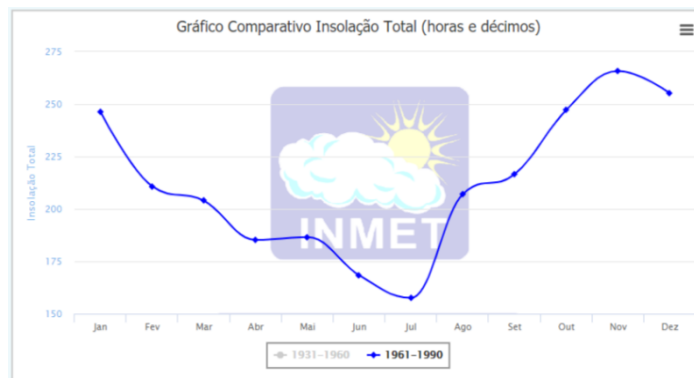
Figura 27 – Gráfico Climatológico da insolação total em Recife – período de 1961-1990
