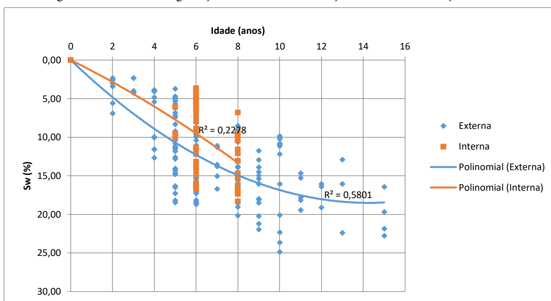
Figura 56 - Curvas de degradação das fachadas em função da influência da ação vento-chuva
