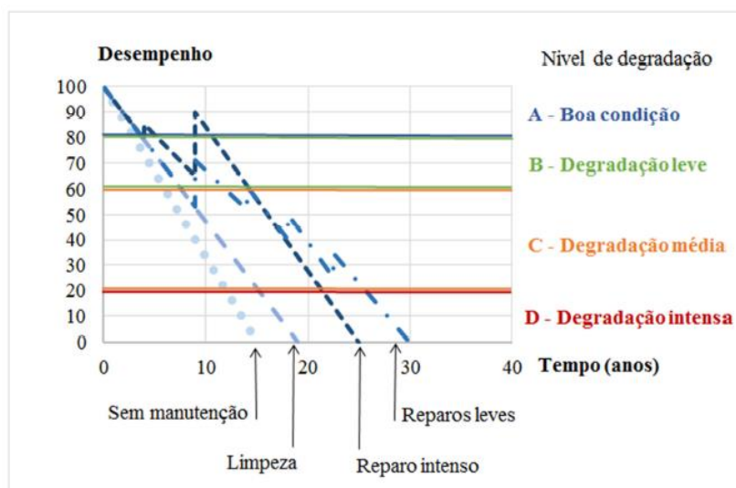
Figura 6 – Relação entre estado de degradação e operação de manutenção em fachadas
