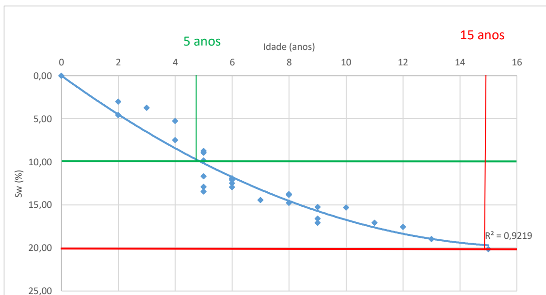
Figura 58 – Curvas de degradação (regressão polinomial) dos 28 edifícios analisados
