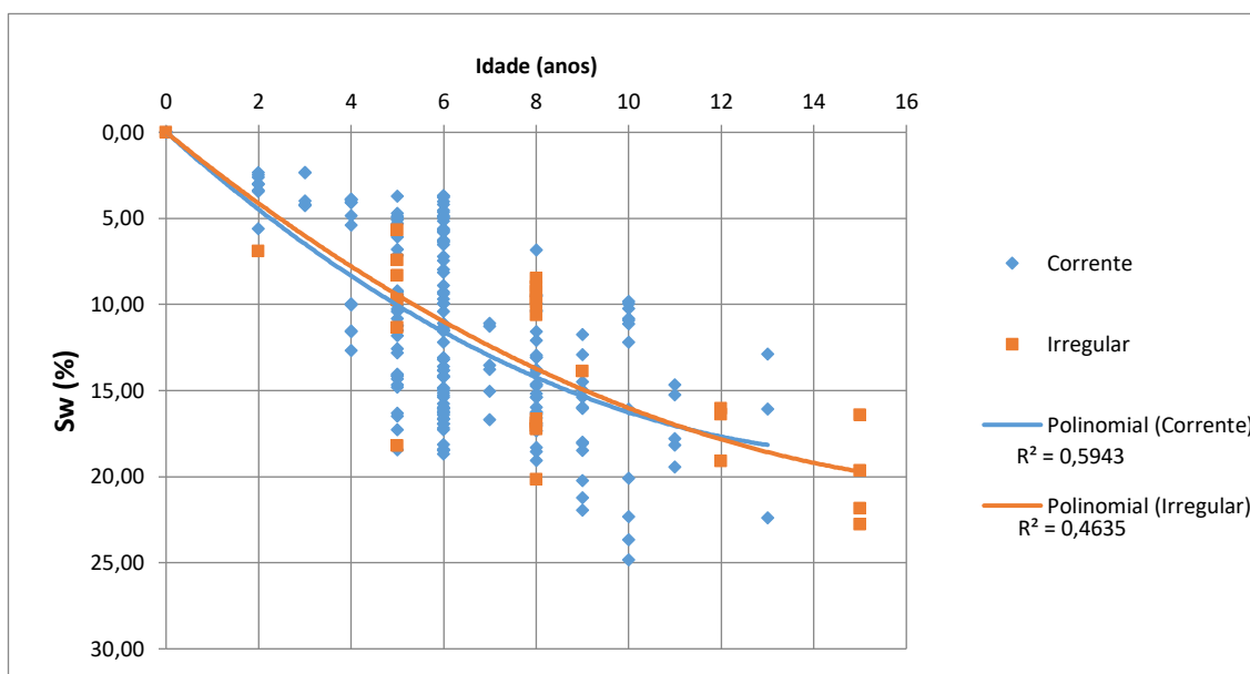
Figura 51 - Curvas de degradação das fachadas em função da geometria
