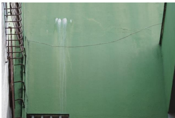
Foto 2 – Exemplo de eflorescência
