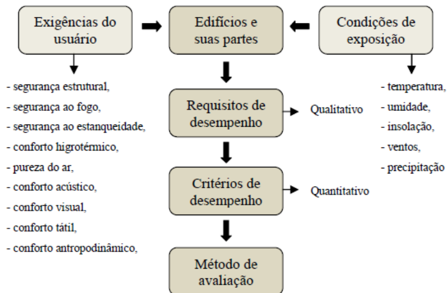
Figura 2 – Metodologia de avaliação de desempenho
