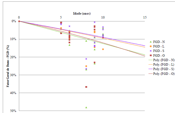
Figura 12 – Curvas de degradação em função da orientação para o Fator Geral de Danos
