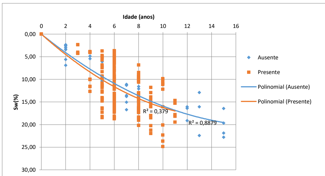
Figura 50 - Curvas de degradação das fachadas em função da presença de detalhes construtivos
