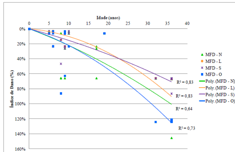
Figura 14 – Curvas de degradação em função da orientação para o Método Fatorial de Danos
