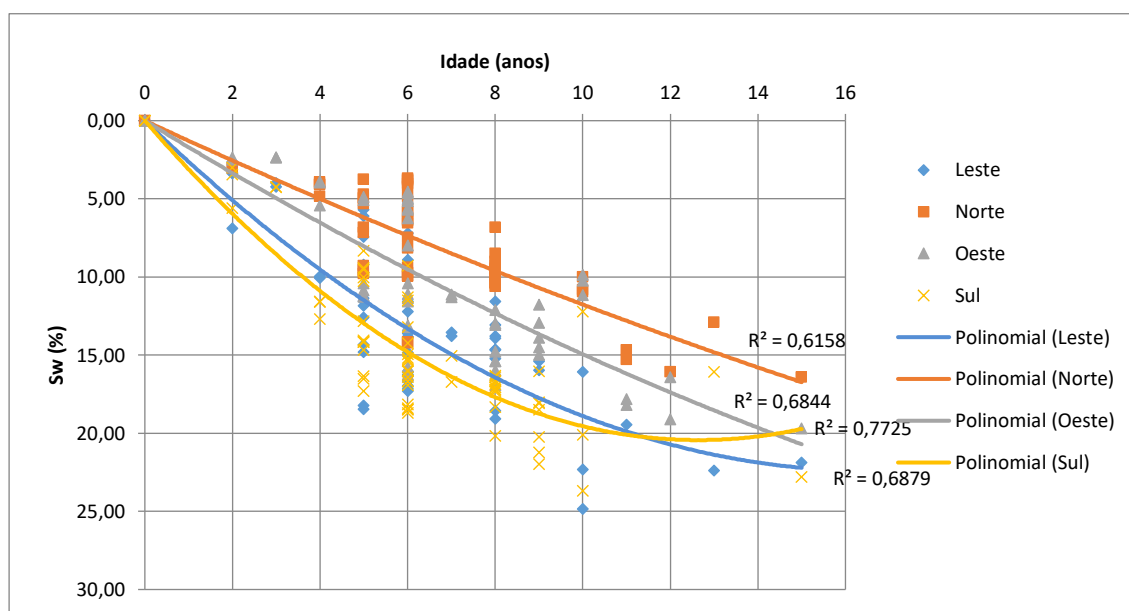
Figura 46 – Curvas de degradação das fachadas analisadas em função da orientação
