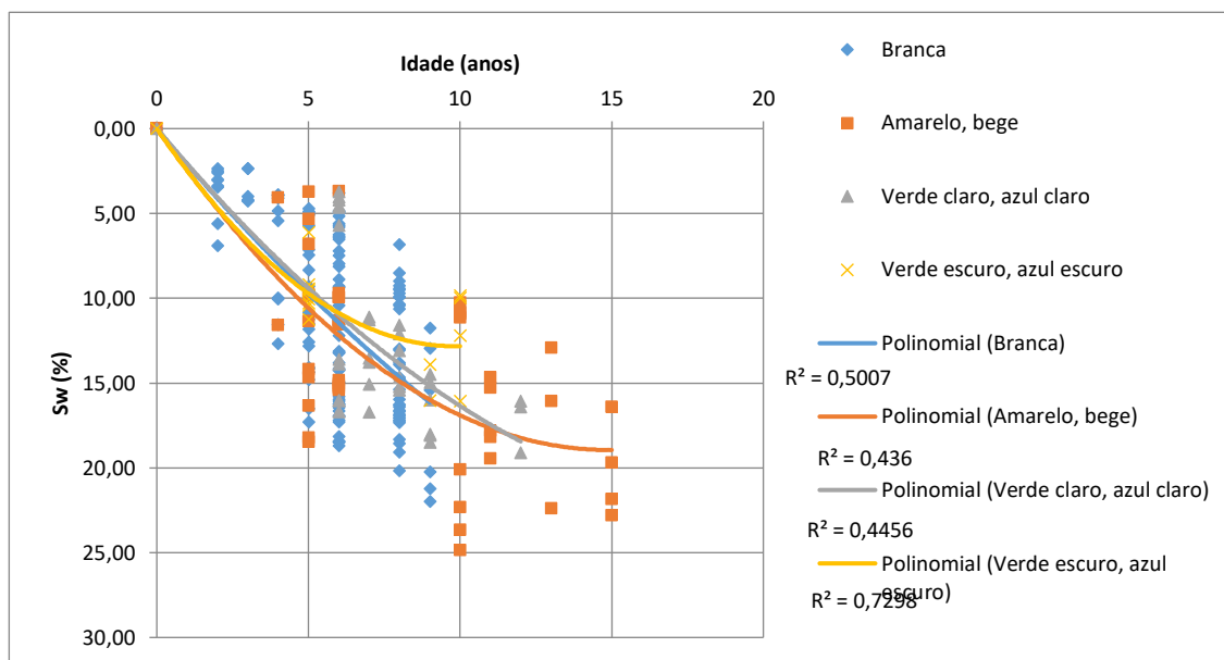
Figura 47 – Curvas de degradação das fachadas analisadas em função da cor
