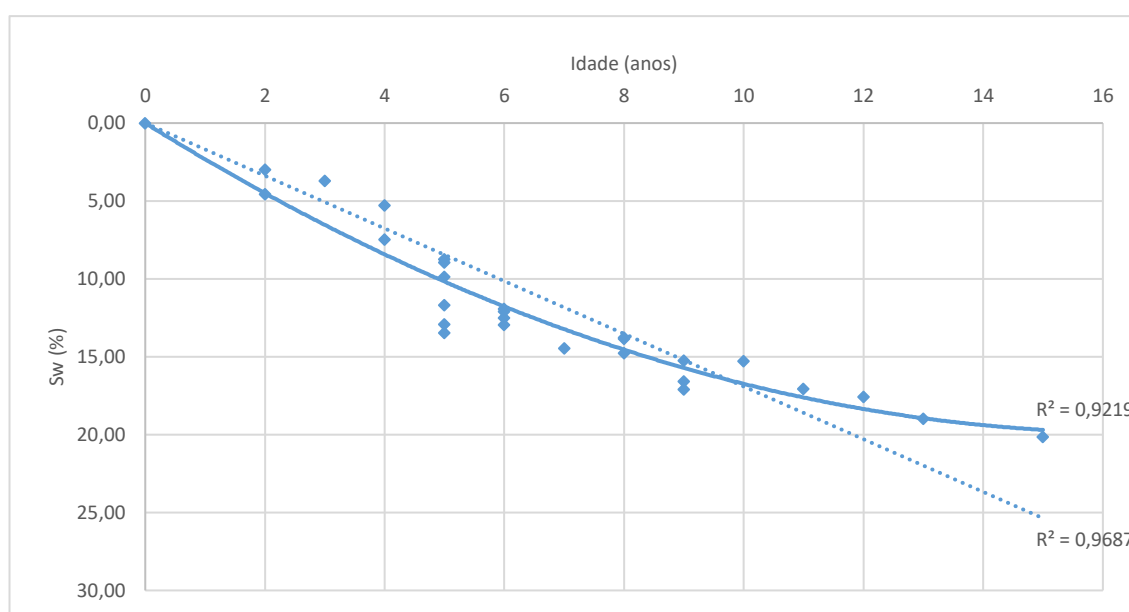
Figura 45 - Curvas de degradação (linear e polinomial) dos 28 edifícios analisados
