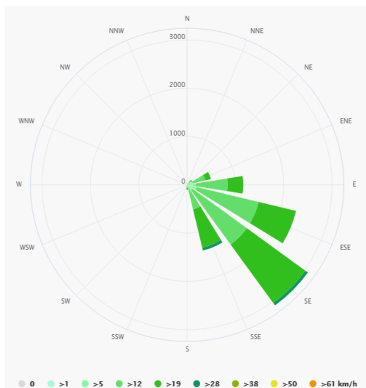
Figura 29 – Rosa dos ventos para Recife apresentando quantas horas por ano o vento sopra na direção indicada
