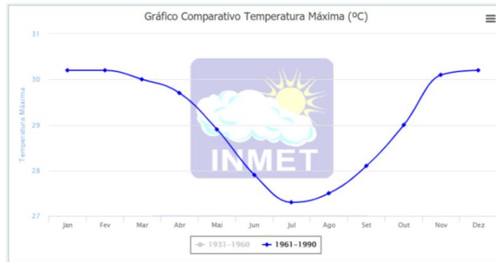
Figura 23 – Gráfico Climatológico da temperatura máxima de Recife – período de 1961-1990
