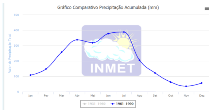
Figura 22 – Gráfico Climatológico da precipitação acumulada de Recife – período de 1961-1990
