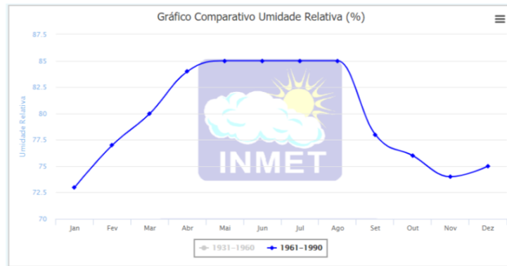
Figura 26 – Gráfico Climatológico da umidade relativa de Recife – período de 1961-1990
