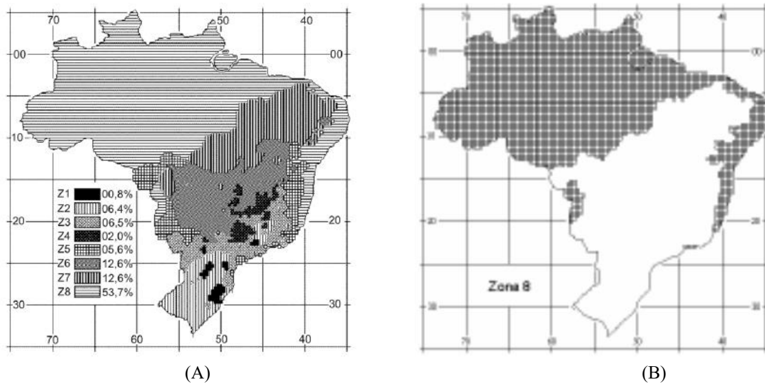
Figura 21 – (A) Mapa de zoneamento bioclimático brasileiro e (B) Mapa com destaque à zona 8 onde se enquadra Recife-PE
