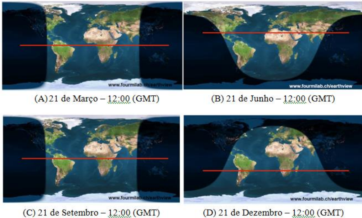
Figura 30 – Vista das áreas sombreadas e ensolaradas da Terra em quatro dias do ano
