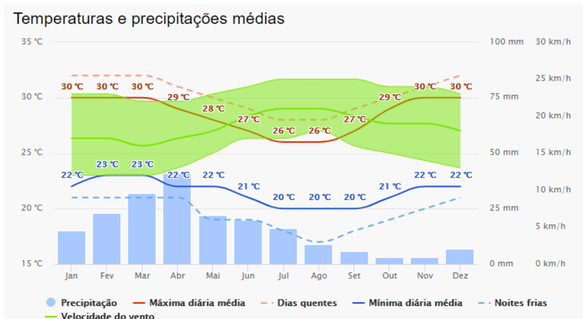
Figura 28 – Gráfico resumo das características climáticas de Recife
