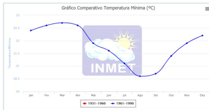
Figura 24 – Gráfico Climatológico da temperatura mínima de Recife – período de 1961-1990
