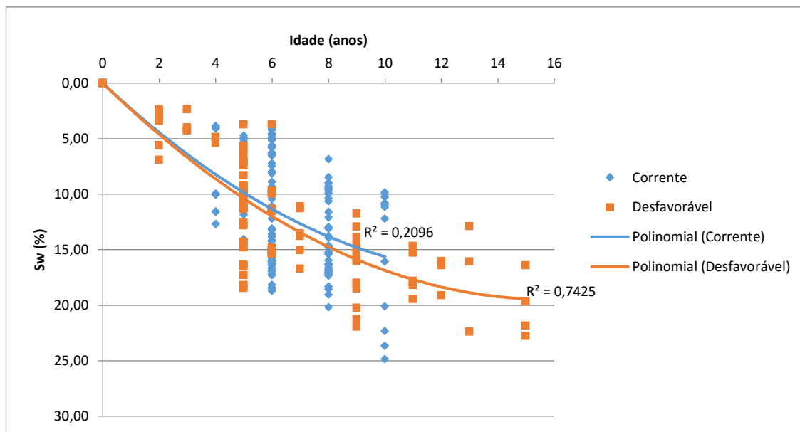
Figura 54 - Curvas de degradação das fachadas em função da proximidade de fontes poluentes
