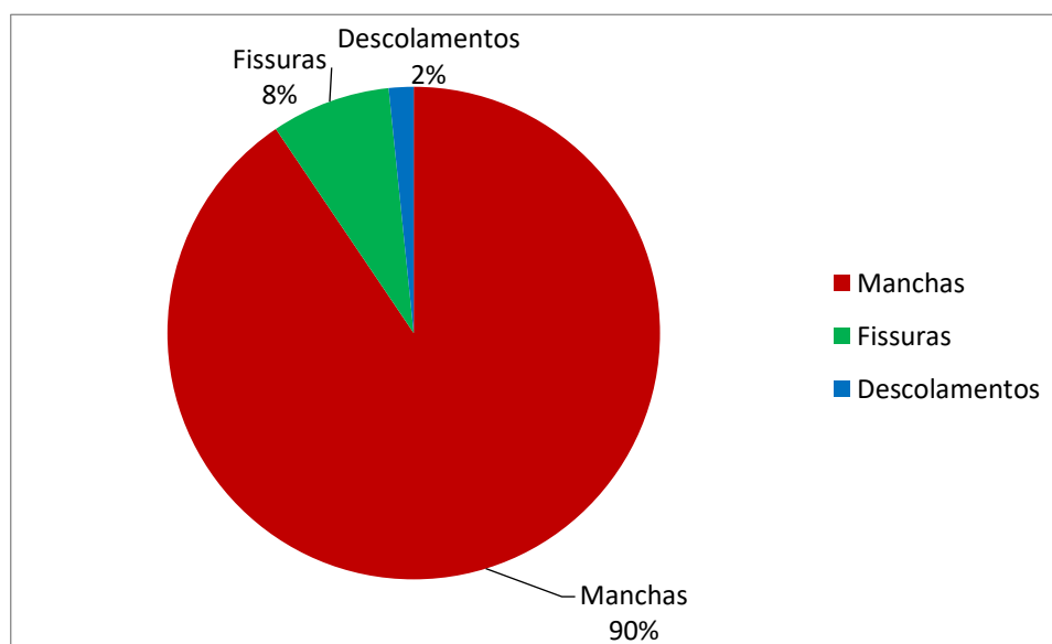
Figura 43 – Ocorrência das patologias nas amostras analisadas
