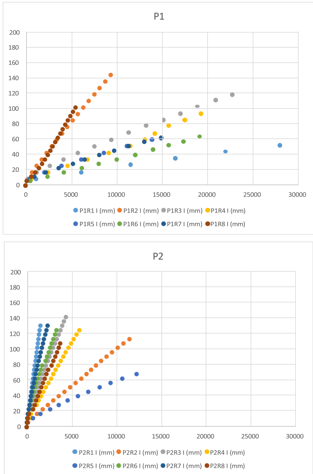
Figura 8 - Curvas de infiltração acumulada em função do tempo para os oitos ensaios realizados.
