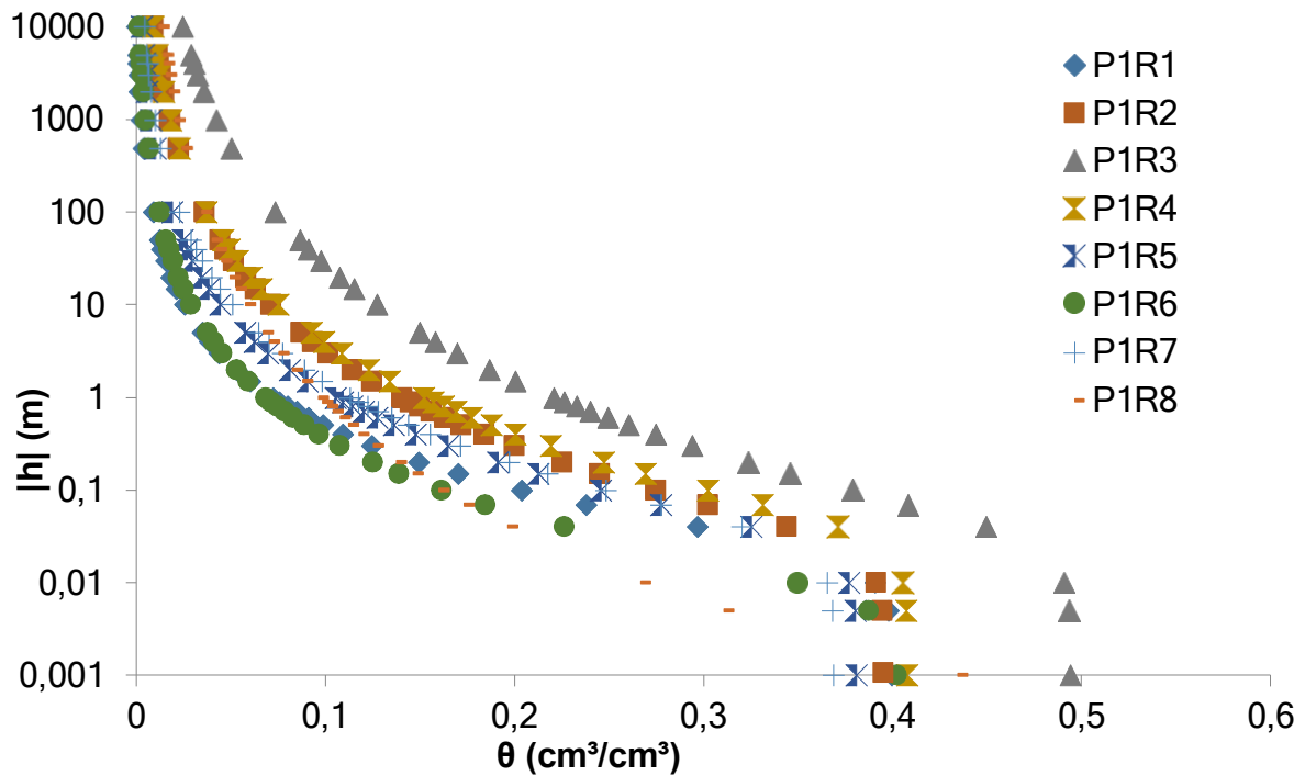
Figura 10 - Curvas de retenção para os ensaios realizados no Parque da Jaqueira.
