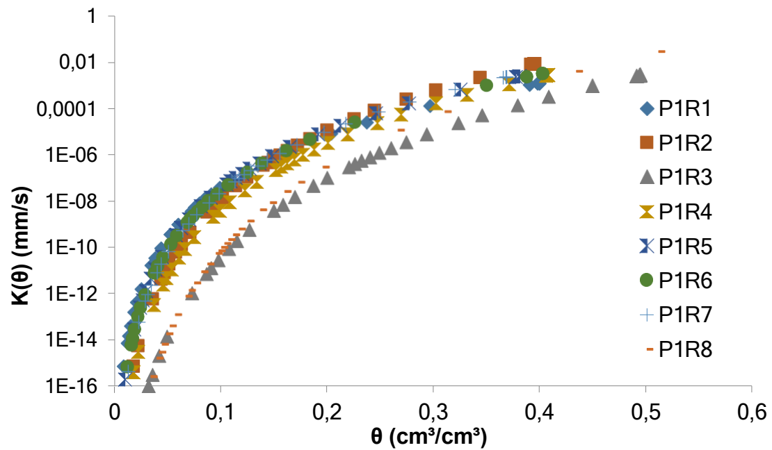
Figura 11 – Curvas de condutividade hidráulica para os ensaios realizados no Parque da Jaqueira.
