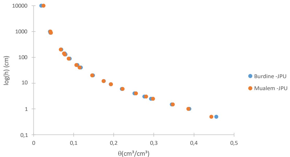
Figura 14 – Ajuste do modelo de distribuição dos poros de Burdine para o modelo de distribuição dos poros de Mualem para as superfícies: Jardim Urbano - JPU, Área de Recreação Infantil - ARI e Área de Convivência – AC.
