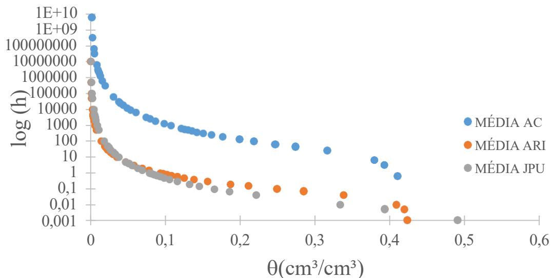
Figura 12 – Curvas de retenção médias para os solos da área de recreação, jardim urbano e área de convivência
